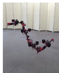
変形飛行ロボット
