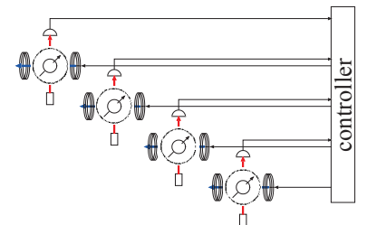
フィードバック制御による多ビット量子スピン系のエンタングルド状態生成
