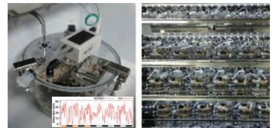
図2 非侵襲睡眠測定装置SSS(左:睡眠測定チャンバー、右:睡眠測定ラック):差圧センサーでチャンバー内の動物の呼吸パターンを自動分類することで睡眠・覚醒リズムを定量的に測定する。
