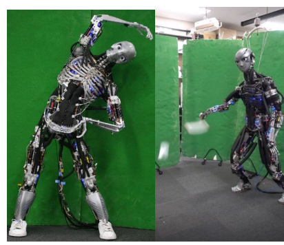
Musculoskeletal robot
